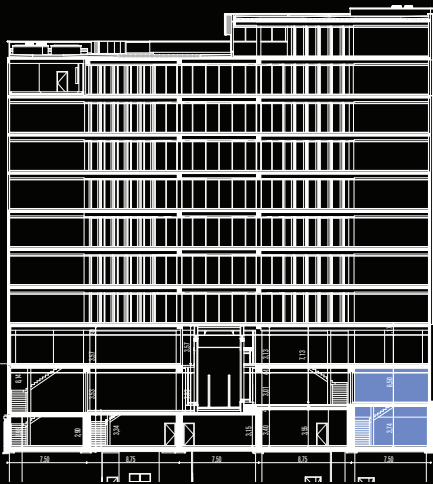
LONGITUDINAL SECTION
