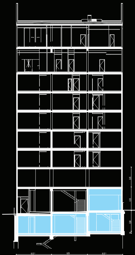
LONGITUDINAL SECTION
